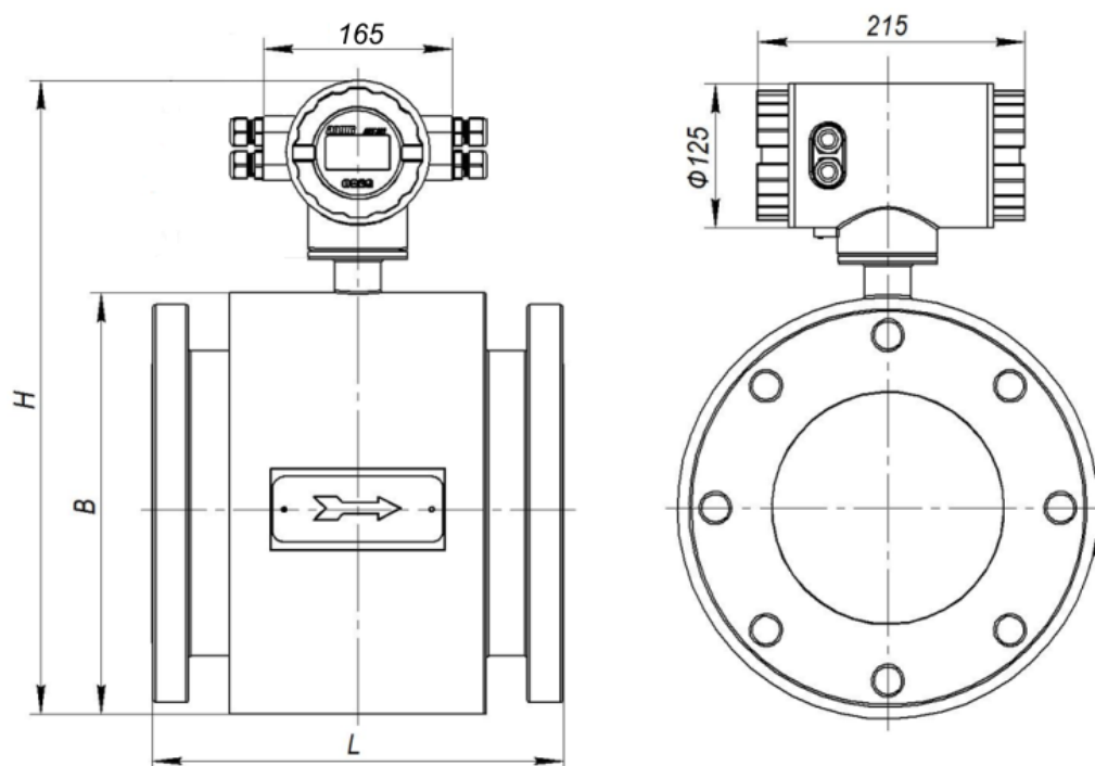
Рисунок А.2 – Габаритные и присоединительные размеры расходомера (Ду ≥ 100 мм)
