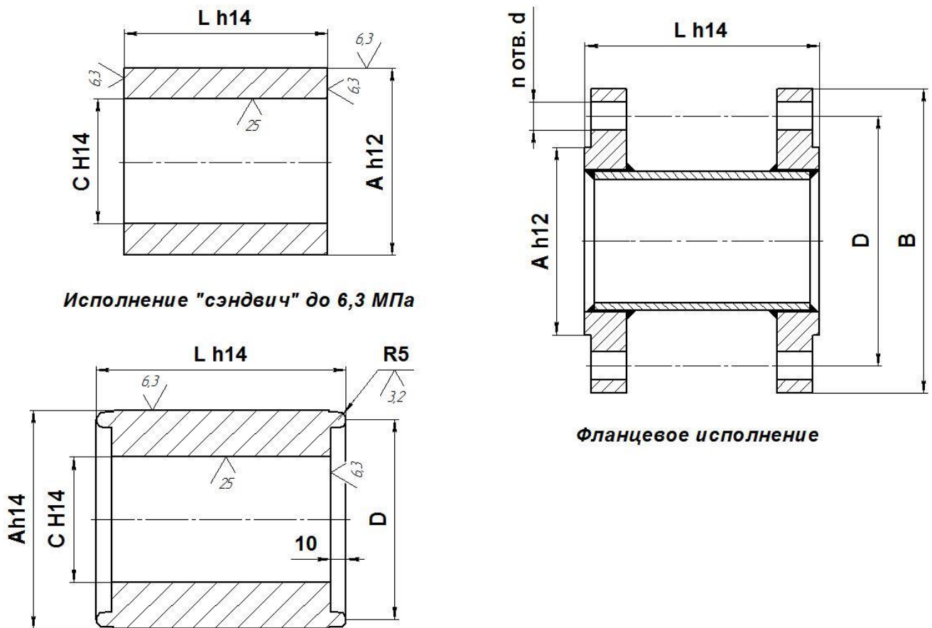
Рисунок В.13 - Размеры преобразователей дистанционного исполнения. Остальные размеры см. Рис. В.3 - В.12
