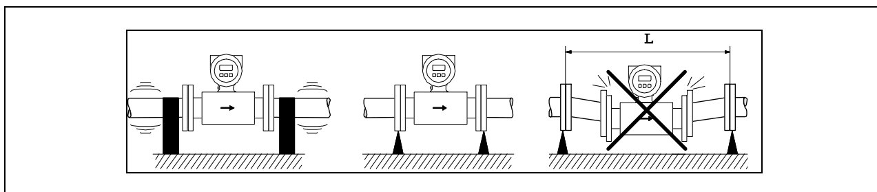
Рис. 13: Меры по предотвращению вибрации измерительного устройства ( L > 10 \text{ м} )
