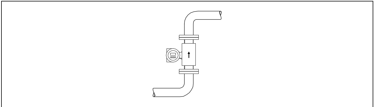
Рис. 9: Вертикальное расположение
