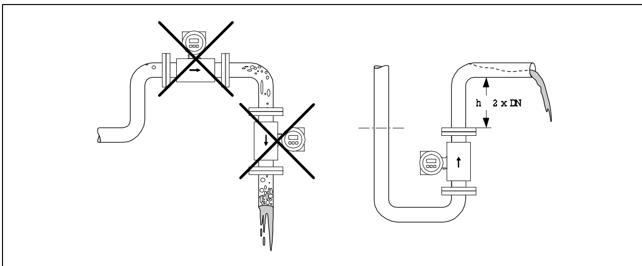
Рис. 6: Место монтажа
