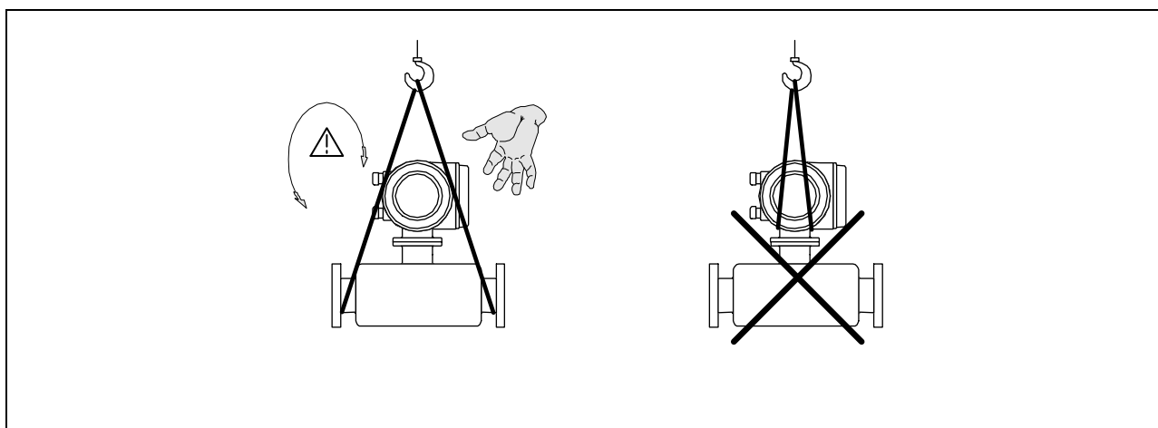
Рис. 4: Транспортировка преобразователя с DN ≤ 300/12"
