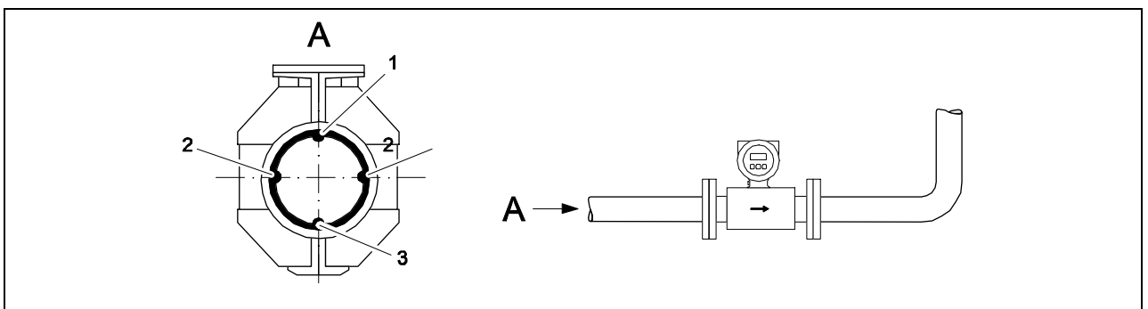
Рис 11: Горизонтальное расположение
