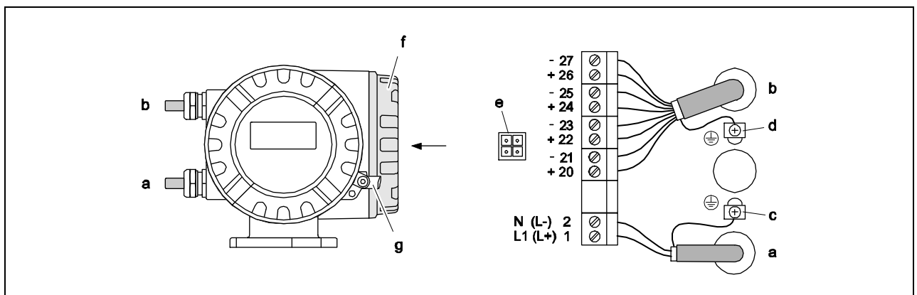
Рис. 27: Подсоединение преобразователя (в алюминиевом рабочем корпусе) Сечение кабеля: макс. 2.5 мм 2 (14 AWG)
