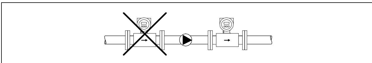
Рис. 7: Монтаж насосов
