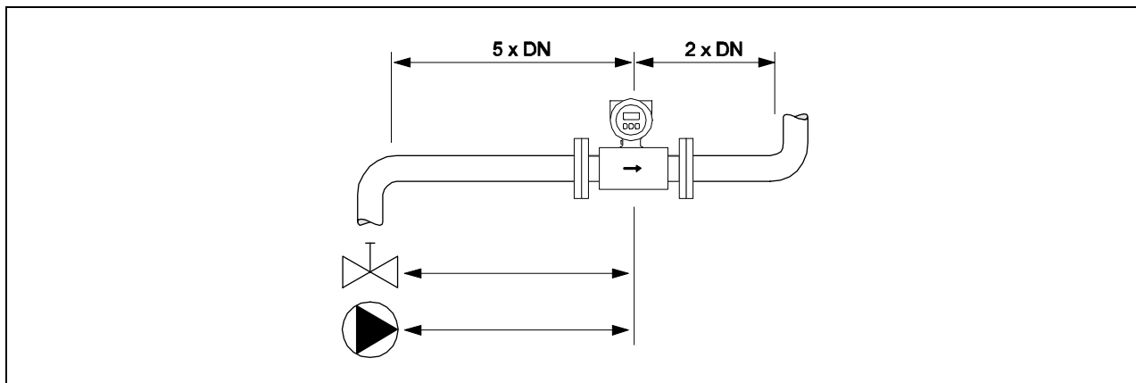
Рис. 12: Входные и выходные участки трубопровода
