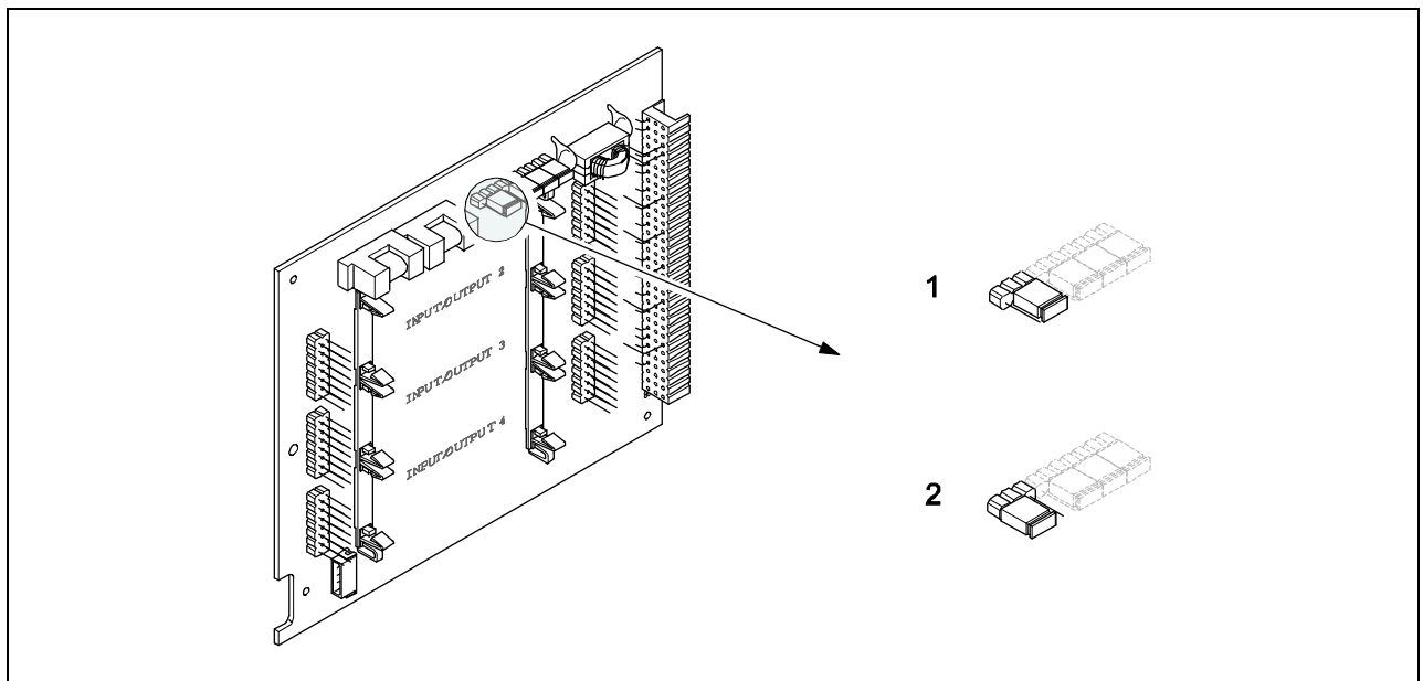
Рис.41: Включение и выключение защиты от записи HART
