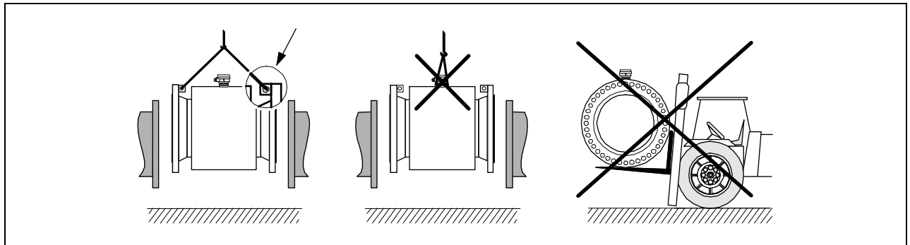
Рис. 5: Транспортировка датчиков с ДУ > 300 (12")
