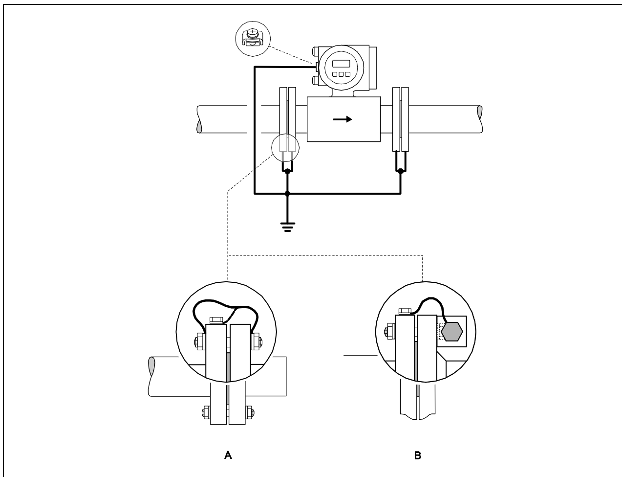
Рис. 32: Выравнивание потенциалов с помощью уравнивающих токов в металлических, незаземленных трубопроводах (заземляющий кабель: медный провод сечением не менее 6 \text{ мм}^2 / 10 \text{ AWG} ).
