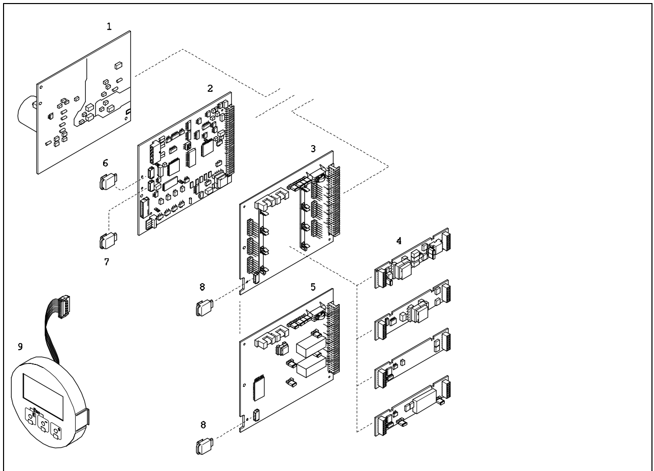
Рис. 54: Корпус настенного блока: снятие и установка печатных плат
